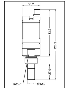
Dimensions FO 510
