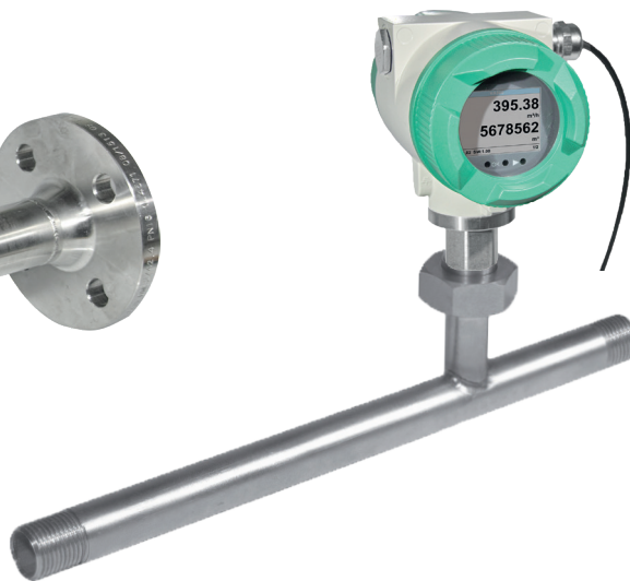
带 R 螺纹或者 NPT 螺纹的版本
