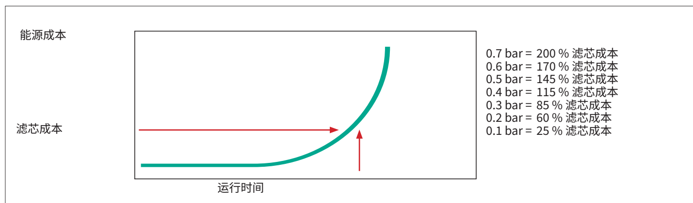
插图:典型的差压曲线,与滤芯成本成比例的能源成本
