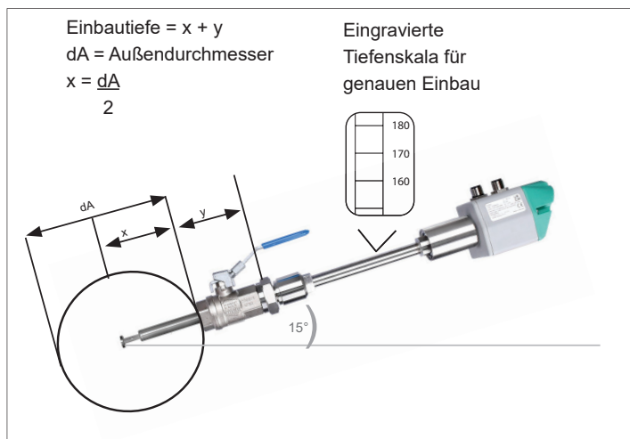
Empfohlene Einbaulage
